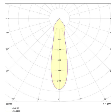
Monza Duo 20°
