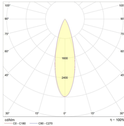
Esen Eco 36°
