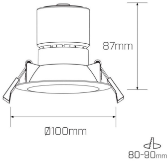
Esen Eco 60°
