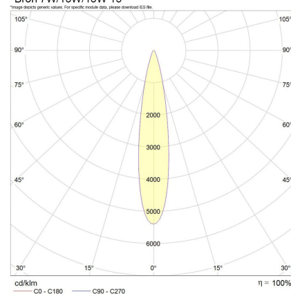
*Bron 7W/13W/18W 15°
