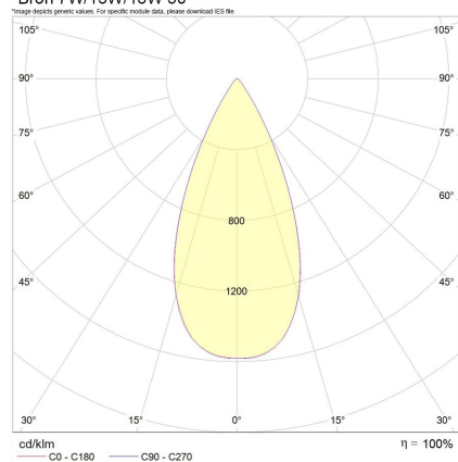
*Bron 7W/13W/18W 50°
