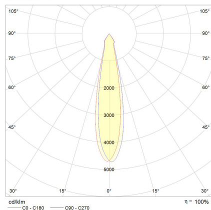
Siena Mini 20°
