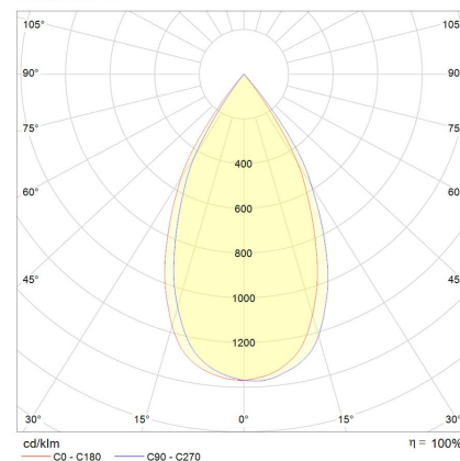
Siena Mini 60°
