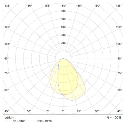
Catania Mini Pendant 17°
