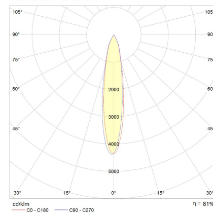
Catania Mini Pendant 20°
